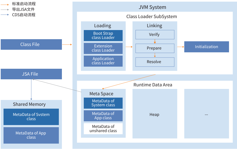
AppCDS 业务流程图
