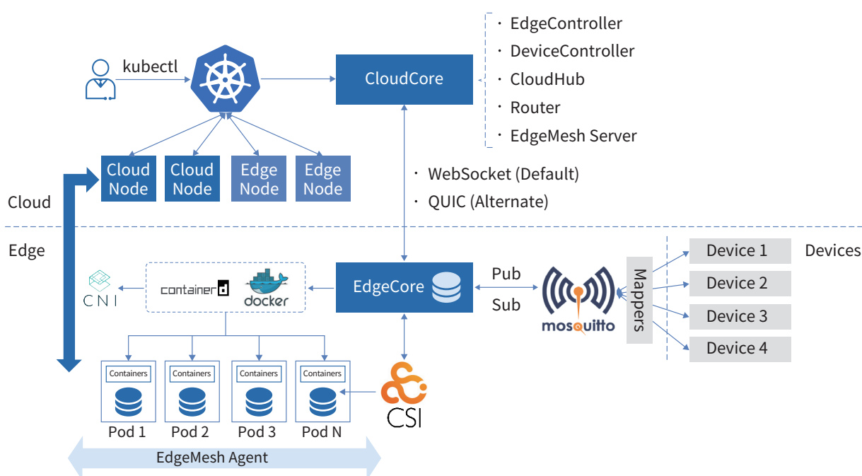
KubeEdge 边云协同基础框架
