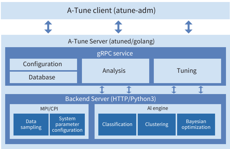
A-Tune 软件架构
