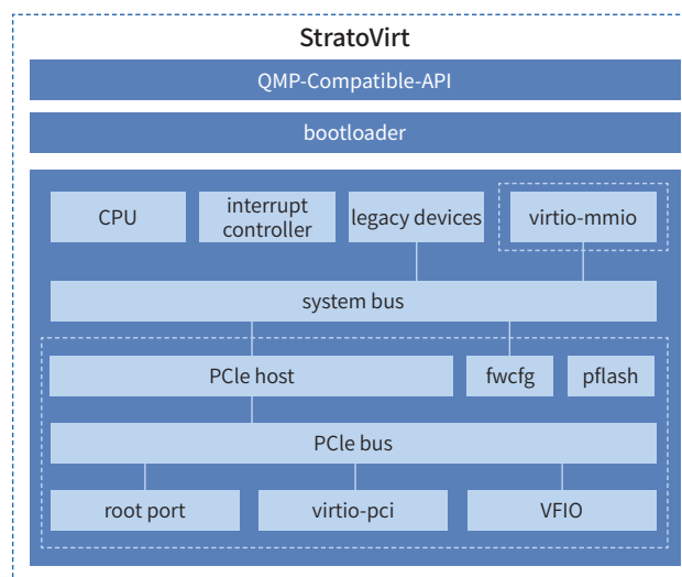
StratoVirt 软件架构
