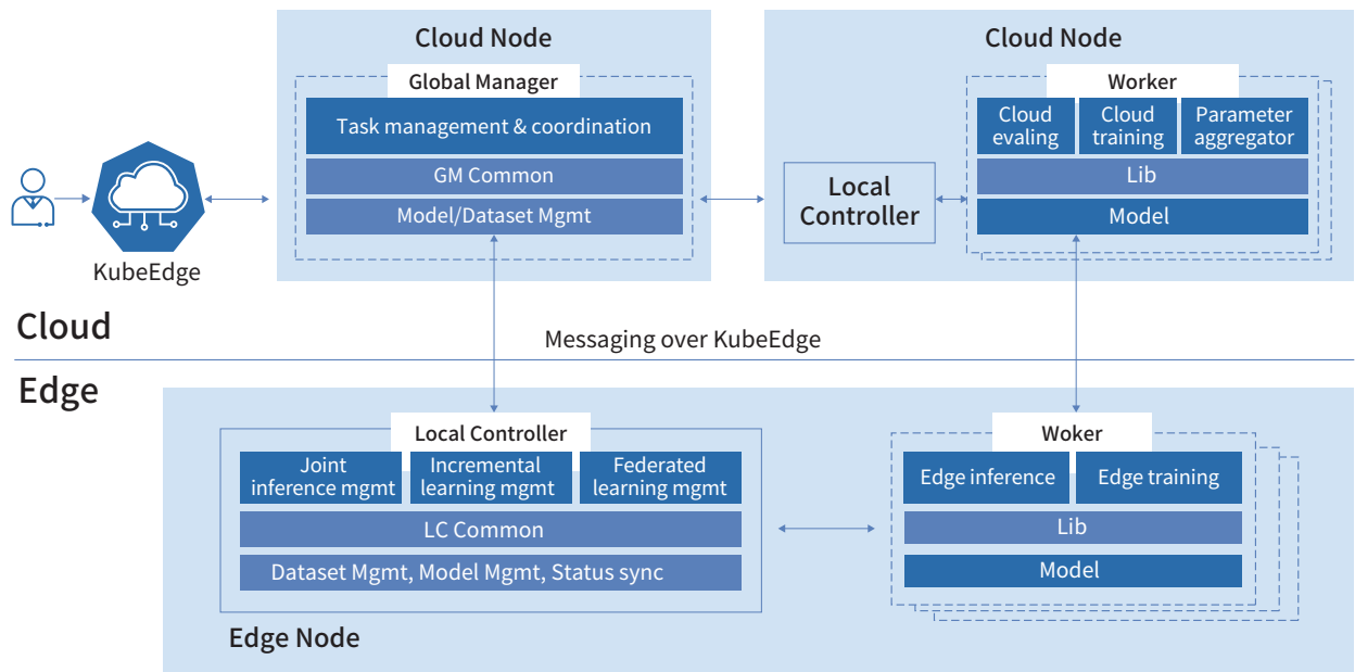
Sedna 边云智能协同框架
