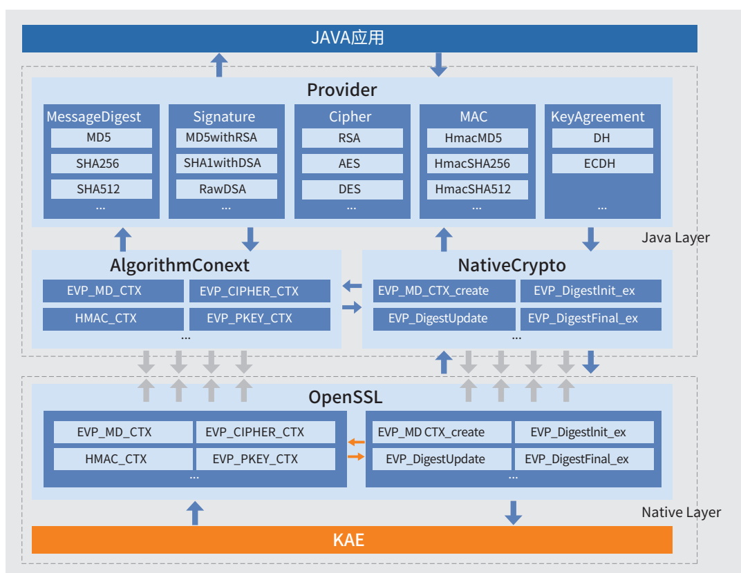
KAE Provider 业务架构图
