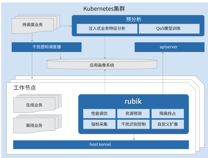
Rubik 混部解决方案
