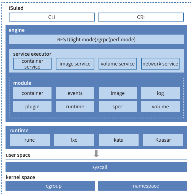
iSulad 软件架构
